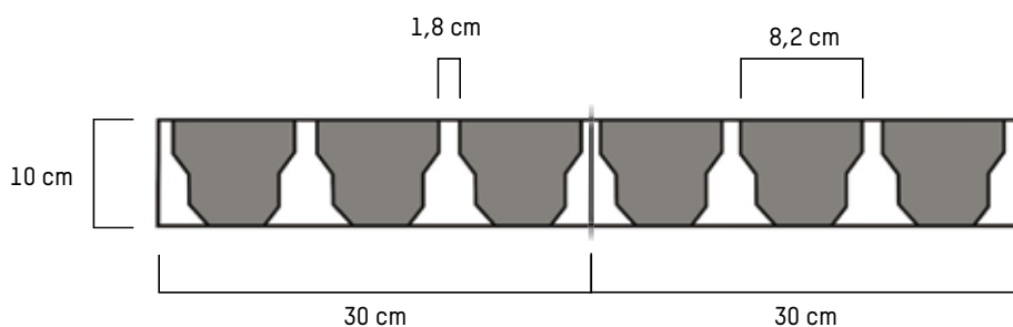
Dostępne: Podłoga szczelinowa o szerokości 30 cm jako element dopasowujący.
