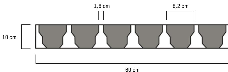
Podłoga szczelinowa dla świń w przekroju
