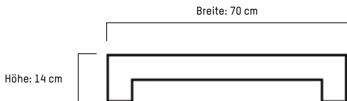
Kotloch-Spaltenboden für Sauen im Querschnitt
