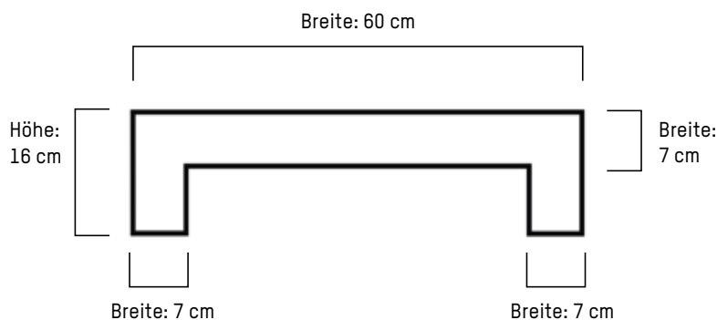
Multirost im Querschnitt
