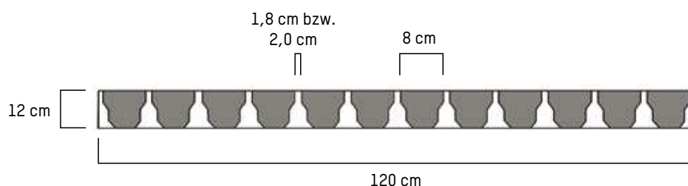
Schweinemast-Spaltenboden im Querschnitt
