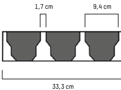
Schweinemast-Spaltenboden im Querschnitt
